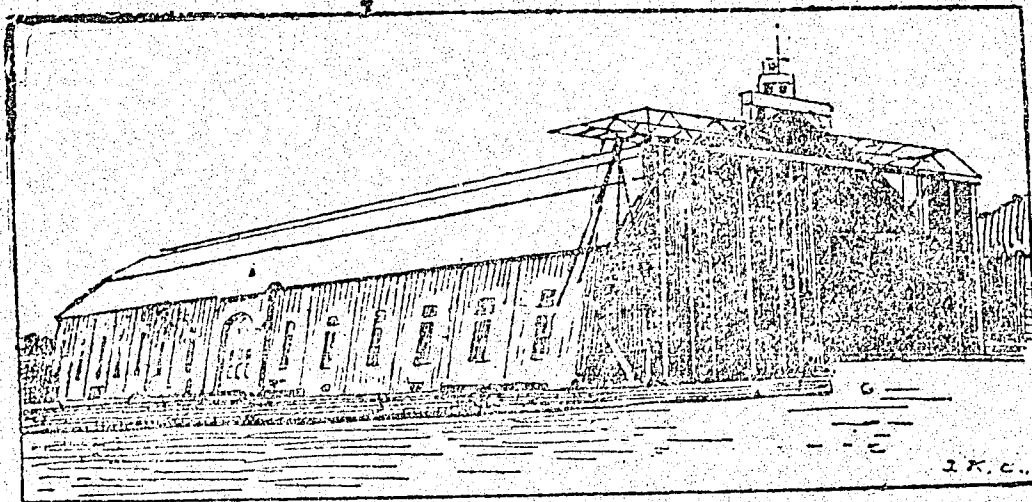
Największa hala na pomieszczenie maszyn lotniczych wybudowana niedawno w Johannisthalu.
